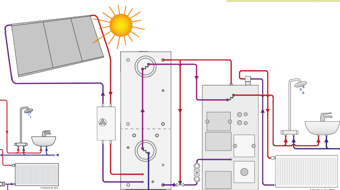
Exempelutförande med solfångare tillsammans med biobränslepanna.
