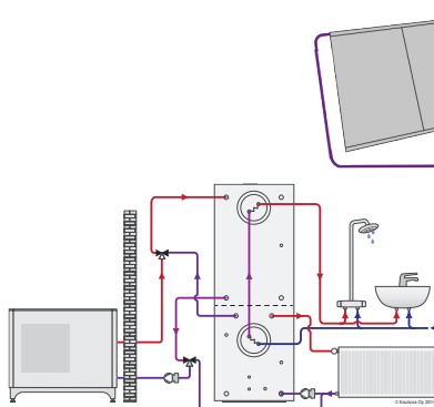
Exempelutförande luft/vatten-värmepump
