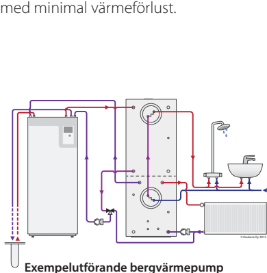
Exempelutförande bergvärmepump
